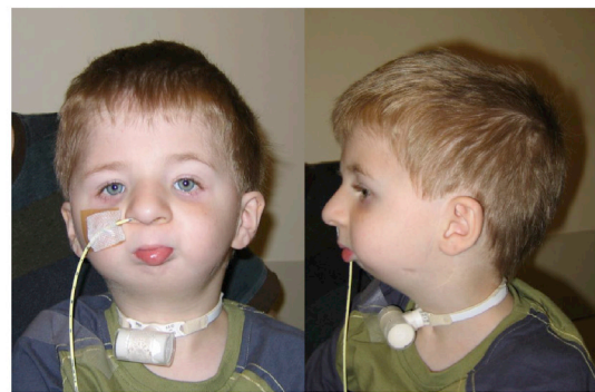
Individual 4 p.(Ala201Val)
